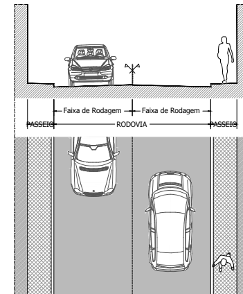
Perfil 03 - passeio + rodovia 2 sentidos + passeio
