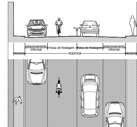
Perfil 03a - passeio + rodovia 2 sentidos c/ estacionamento informal nos 2 sentidos + passeio
