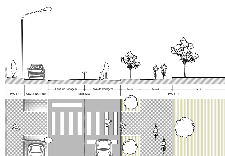
Perfil 07 - passeio + estacionamento + rodovia 2 sentido + jardim + passeio + jardim
