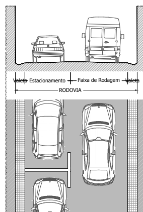
Perfil 04 - estacionamento + rodovia 1 sentido
