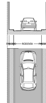
Perfil 05b - passeio + rodovia 1 sentido + passeio
