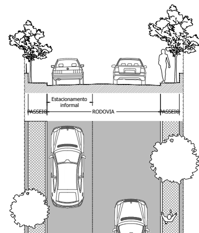
Perfil 05 - passeio + estacionamento informal + rodovia 1 sentido + passeio
