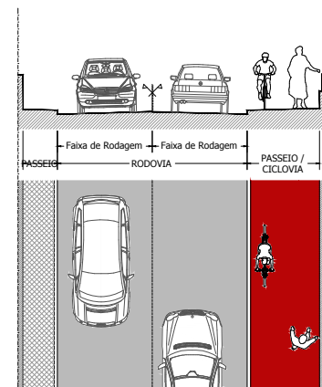
Perfil 02 - passeio + rodovia 2 sentidos + passeio / ciclovia 2 sentidos partilhada
