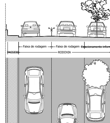
Perfil 05a - passeio + rodovia 2 sentidos + estacionamento informal
