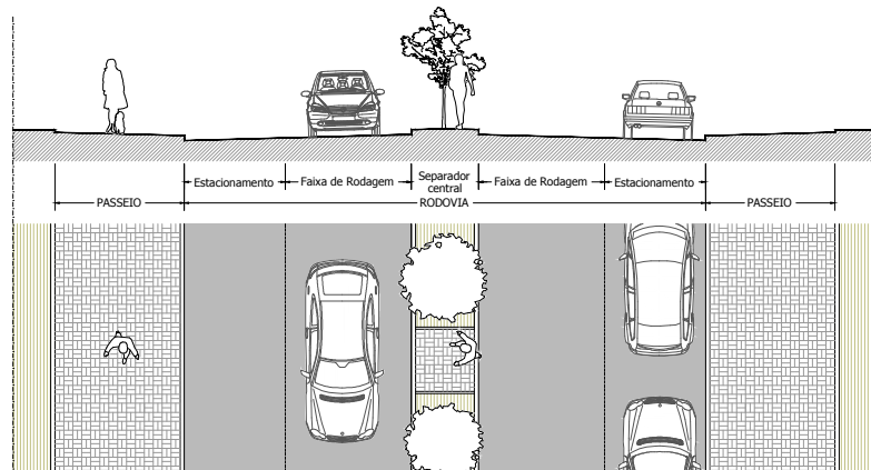
Perfil 06a - passeio + rodovia 2 sentidos c/ separador central + passeio
