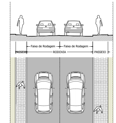
Perfil 03b - passeio + rodovia 1 sentido, 2 faixas + passeio
