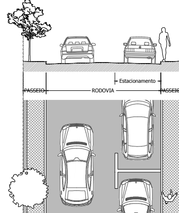
Perfil 04a - passeio + rodovia 1 sentido + estacionamento + passeio
