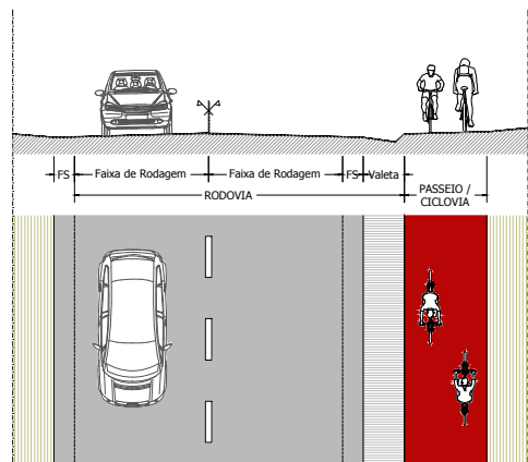
Perfil 01 - rodovia 2 sentidos + ciclovia 2 sentidos partilhada com o peão
