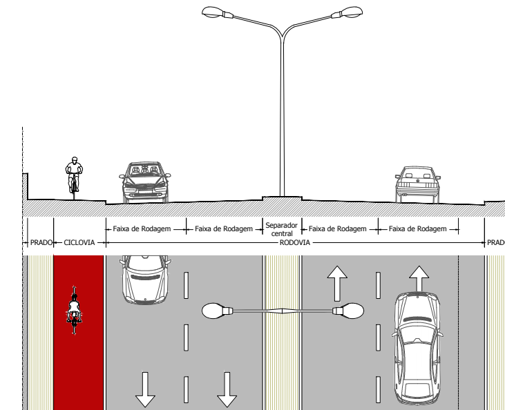
Perfil 06 - ciclovia + rodovia 2 sentido, 2 faixas + faixa de segurança
